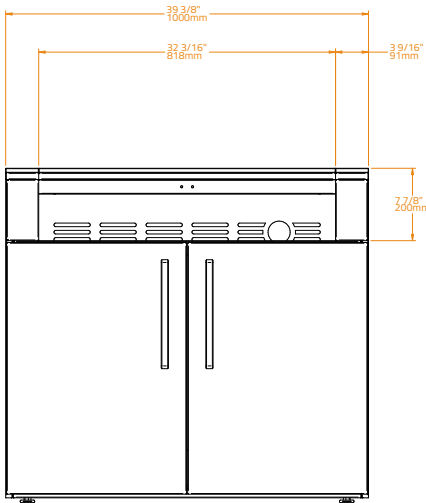
KC 100 Plancha KC 100 Skříňka pod plancha gril Kód BKC0023
