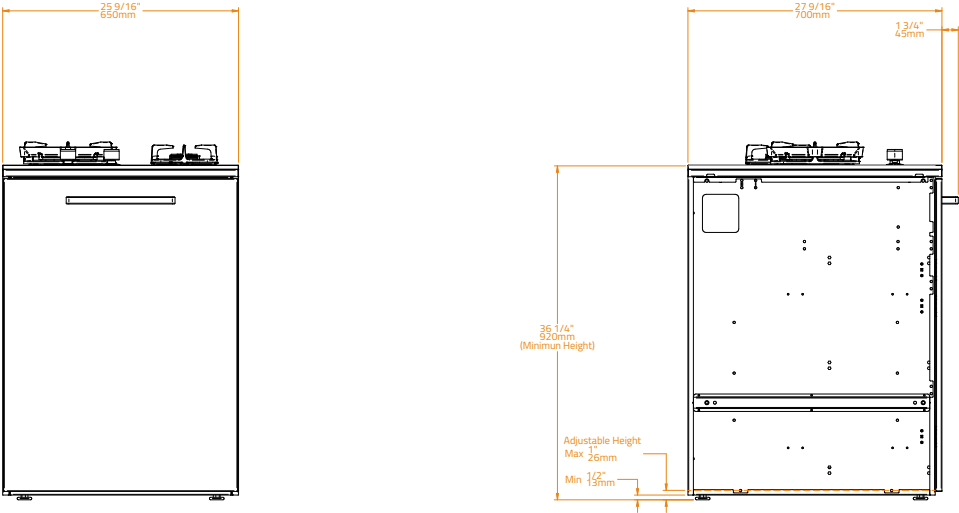
CT 60 Countertop Side Burners CT 60 Skříňka s hořáky Kód BKC0025
