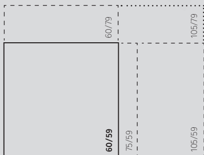
Rozměry prosklení: plynové krby s Prestige hořákem (GP řada)
