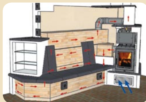
... mit Heizwasser-Aufsatzregister (für die Anbindung an das Heizungssystem) und keramischem Zug.
