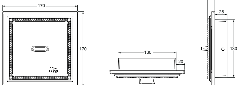
Litinová vymetací dvířka
