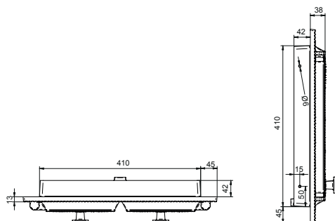
Litinová příkladací a popelníková dvířka se sklem
