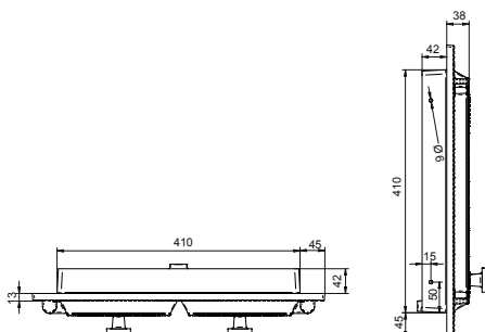
Litinová dvířka se sklem
